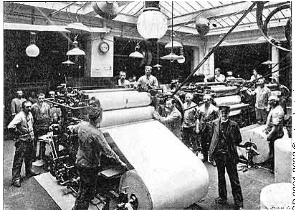
Rotative du Petit Journal 1894
