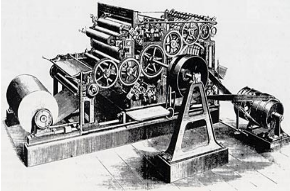
Rotative des années 1870
